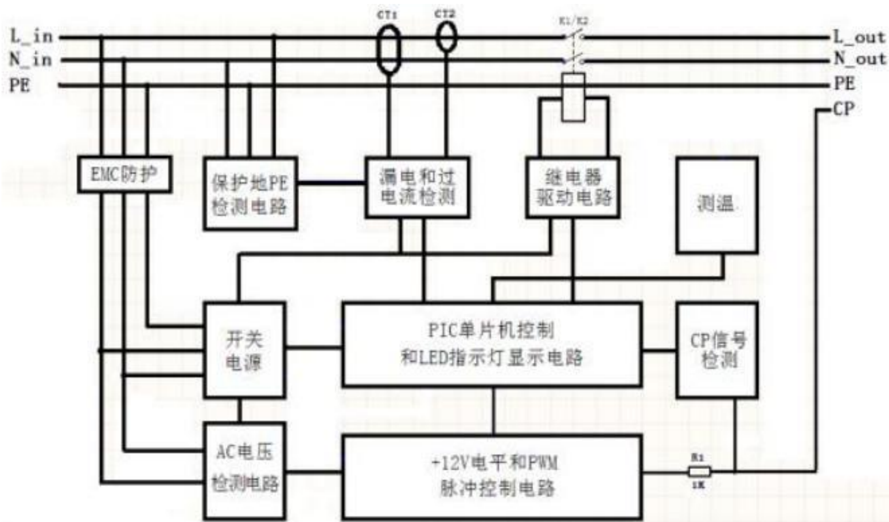
充电盒电气原理图
