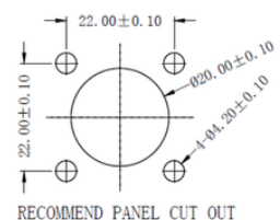
推荐面板安装尺寸
