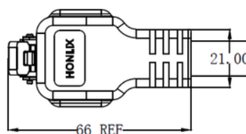
推荐面板安装尺寸
