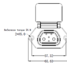
推荐面板安装尺寸
