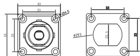
开孔尺寸 Hole Size
