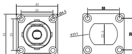
开孔尺寸 Hole Size
