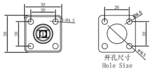
推荐面板安装尺寸
