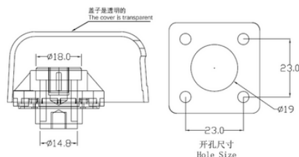
推荐面板安装尺寸
