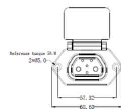
推荐面板安装尺寸
