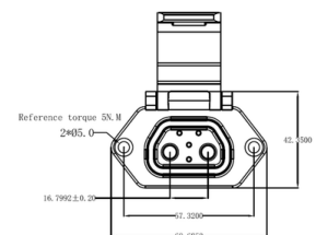
推荐面板安装尺寸
