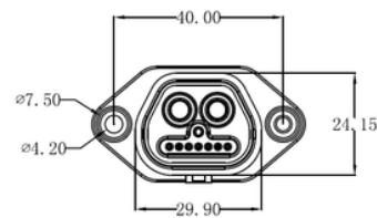
推荐面板安装尺寸
