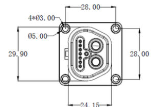
推荐面板安装尺寸
