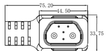
推荐面板安装尺寸
