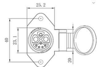
推荐面板安装尺寸
