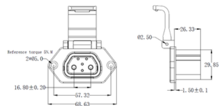
推荐面板安装尺寸
