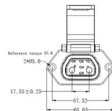
推荐面板安装尺寸
